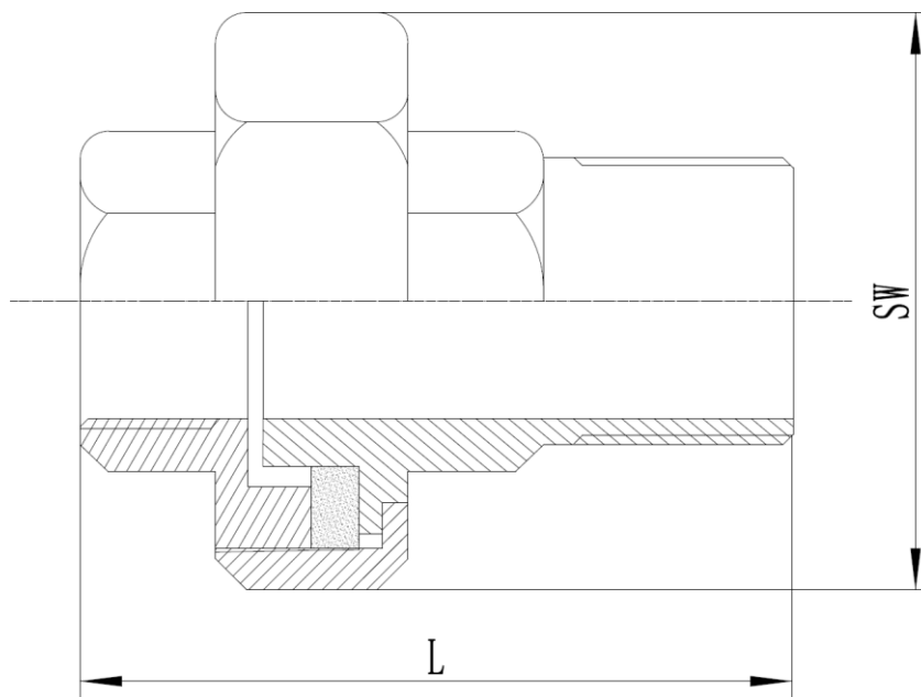
311A Verschraubung flach dichtend, Innen-/Außengewinde Union, flat seat, female / male thread, V4A / AISI 316
