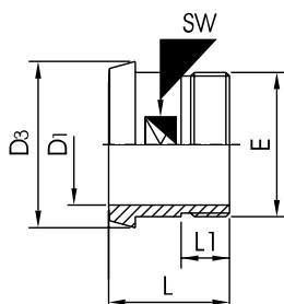
Kegel-Einschraubstutzen
