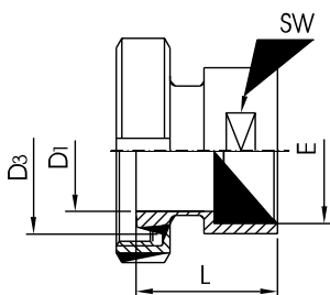
Kegel-Aufschraubstutzen
