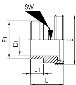
Gewinde-Einschraubstutzen
